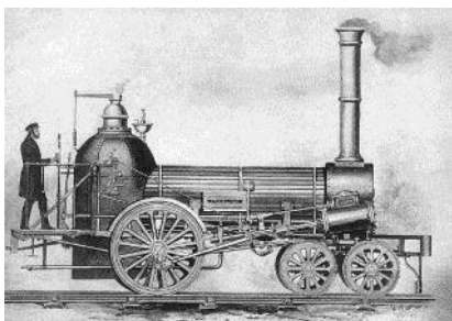
Levo lokomotiva Norris - George Washington s kolesnim razporedom 4-2-0 (osni razpored 2'A) iz leta 1836 in desno Norris - Virginia s kolesnim razporedom 4-4-0 (osni razpored 2'B) iz leta 1842. Ta je bila osnova za načrtovanje in izdelavo lokomotive Ocean.
